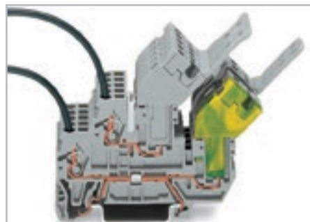
Розетки углового исполнения обеспечивают уменьшение высоты установки
