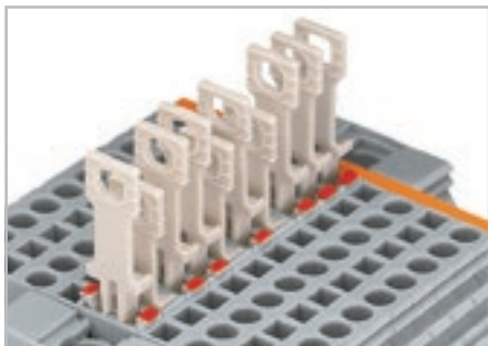
Клемма с размыкателями с цветным стопором для указания состояния переключателя (красный = разъединение)
