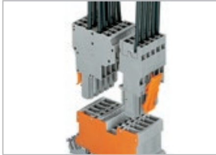
2-контактная экранированная базовая клемма 2-проводная розетка 1-проводная розетка, прямая*
