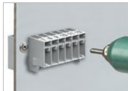
Монтаж с помощью глухих заклепок диаметром 3 мм
