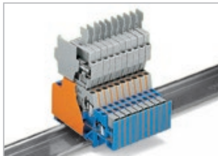
При использовании двухуровневых клемм вместе со штекерами с предохранителями (ширина 6 мм) на уровне розетки (верхний), превышенная длина может быть компенсирована для серии 280 (ширина 5 мм) с помощью промежуточной пластины (толщиной 1,1 мм). Если требуется, для такой промежуточной пластины возможно объединение перемычками на нижнем уровне с помощью вставных поперечных перемычек (280-402).
