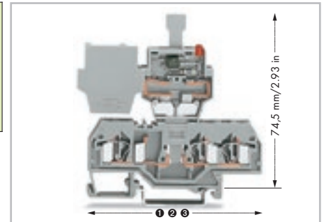
Размеры базовых клемм с штекерным предохранителем
