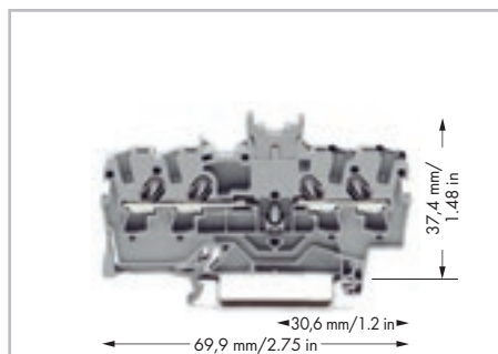
Двухпотенциальные клеммы с двойным маркировочным разъемом в центре клеммы, серые 2001-1441 В упаковке: 100 шт
