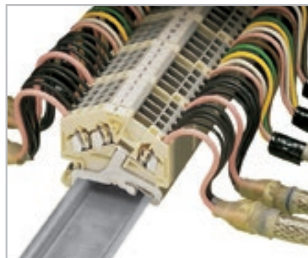
Пример применения для экранированных клемм
