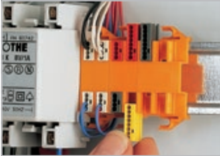
Установка клемм PUSH WIRE® для распределительных коробок в держатель.
