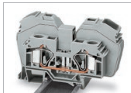
Клеммы серии 285 могут объединяться с клеммами серии 283: 285-635 или 285-634 с 283-601 или 283-604
