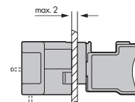
Штекер-розетка с боковым фиксирующим рычагом
