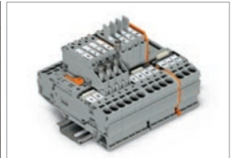
Поворотный держатель предохранителя с запасными патронами
