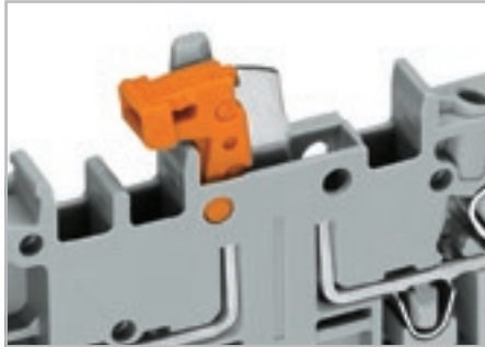
2-проводная клемма с размыкателем для тестирования и измерений с ножевым размыкателем и механическим фиксатором Разомкнутое положение
