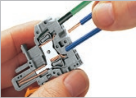
Розетка: подсоединение/отсоединение проводника. Возможен также монтаж под углом в 90°.
