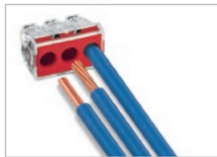
Подключение одножильных и многожильных проводников 6 мм²/AWG 10.
