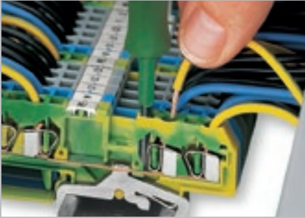
Зажим проводника
