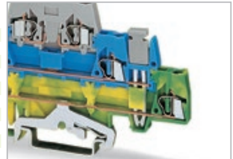
Заземление на несущую DIN-рейку. Подключение N-уровня к уровню заземления с помощью вертикальной перемычки
