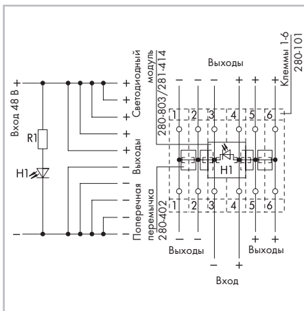
Несколько выходов с индикаторной лампочкой
