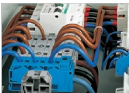
Распределительные клеммы, монтируемые на рейку с соединением винтовым зажимом 35 мм 2 /AWG 2 (фронтальный вход) и соединением 3 x 10 мм 2 /AWG 8 CAGE CLAMP® с фронтальным входом. Для монтажа на несущие рейки DIN 35 согласно EN 60675. Клемма закрыта с обеих сторон, торцевая или промежуточная пластина не требуется.
