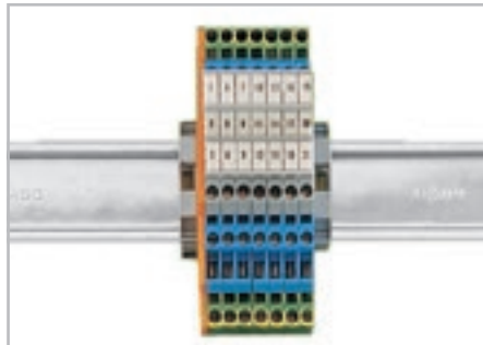
Двух (трех-) уровневые клеммы содержат две (три) независимые шины; в серии 280 уровни могут различаться цветовым обозначением. Нижний уровень шире для упрощения прокладки кабеля.
